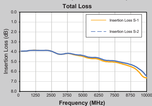
EP2W1+ (500-9500MHz)
