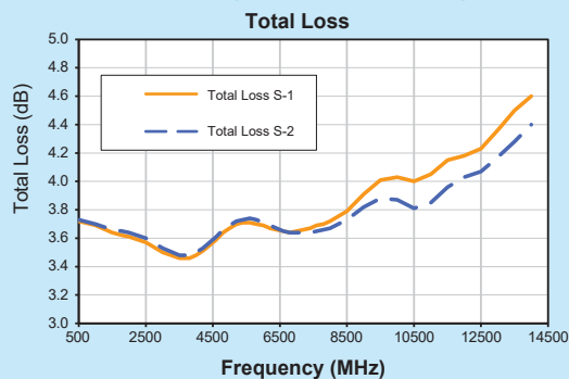
EP2C+ (1800-12500MHz)
